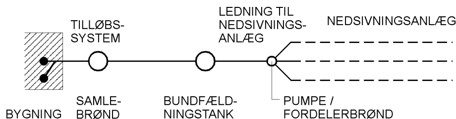
Figur 1.1. Principskitse af et mindre afløbsanlæg med nedsivning.
